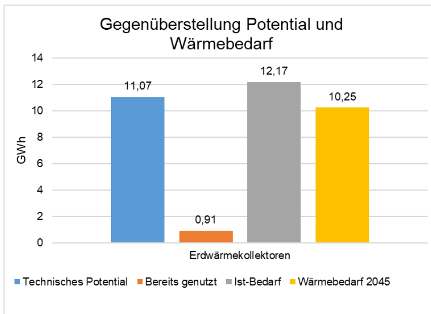
Abbildung 17: Potenzial Erdkollektoren
