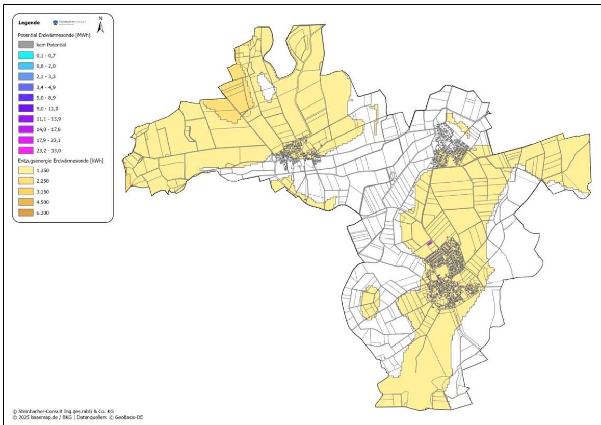
Abbildung 18: Entzugsleistung Erdsonden
