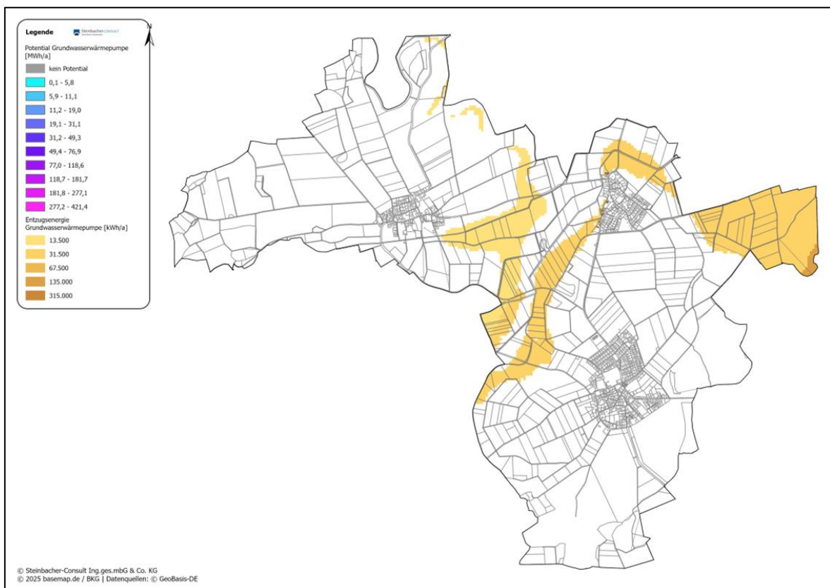
Abbildung 20: Entzugsenergie Grundwasserbrunnen
