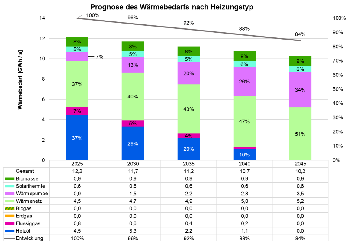
Abbildung 30: Entwicklung Wärmebedarf nach Energieträger
