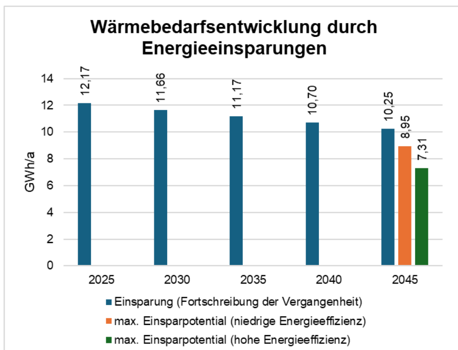
Abbildung 14: Wärmebedarfsentwicklung durch Energieeinsparungen
