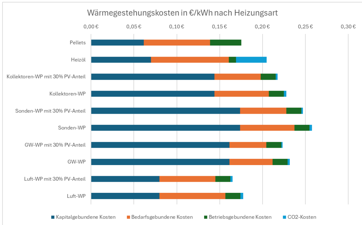
Abbildung 34: Wärmegestehungskosten Wärmeversorgungsarten unsaniertes Einfamilienhaus
