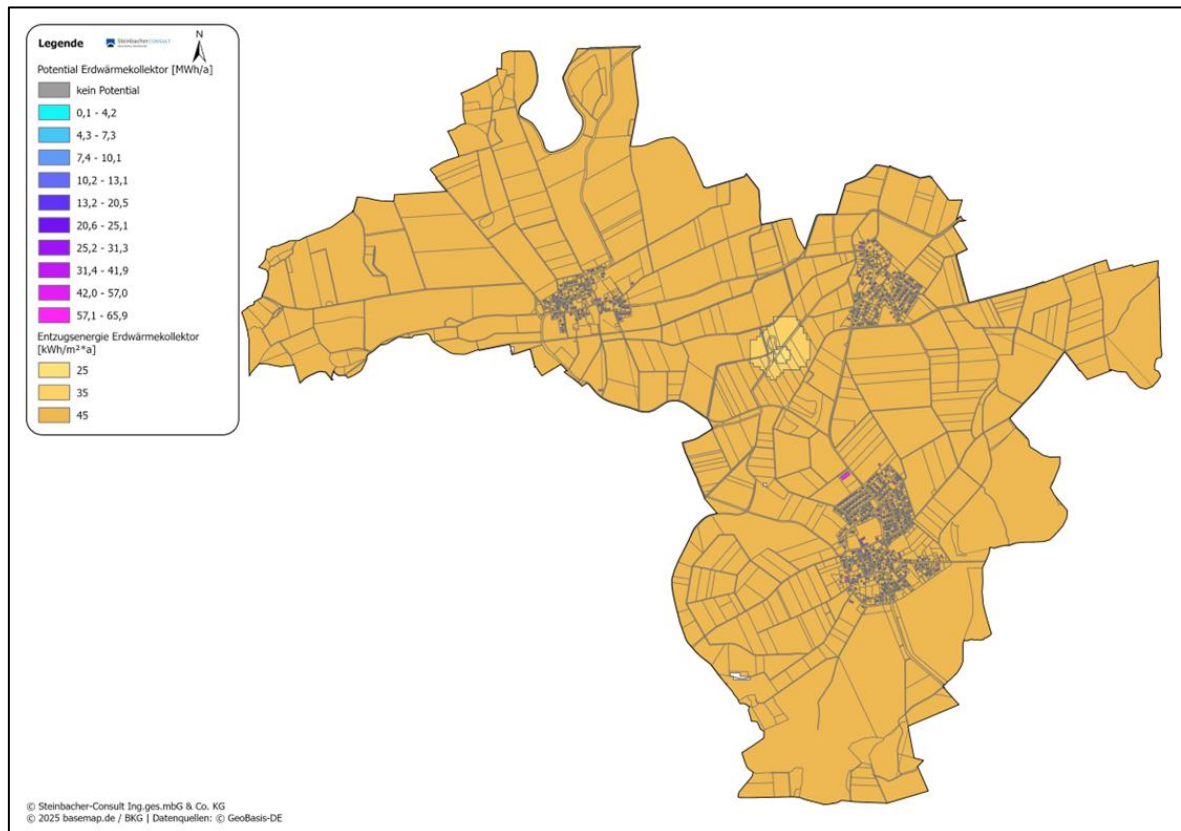
Abbildung 16: Entzugsenergie Erdkollektoren
