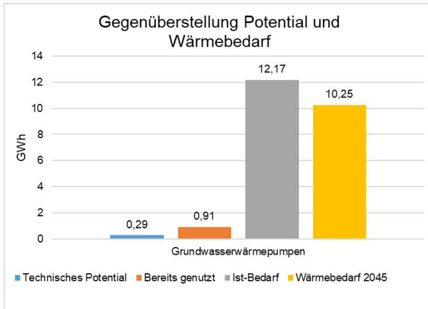
Abbildung 21: Potenzial Grundwasserbrunnen
